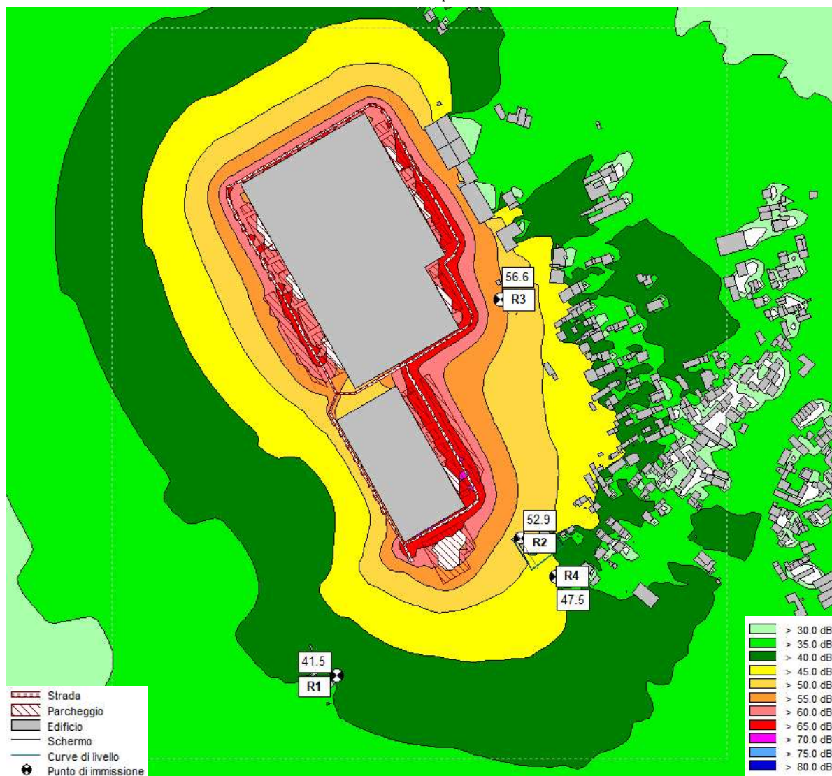
Figura 6-5 – Sorgenti interne - Mappa degli isolivelli acustici DIURNI calcolata a 4 metri di altezza dal suolo – Scenario di punta
