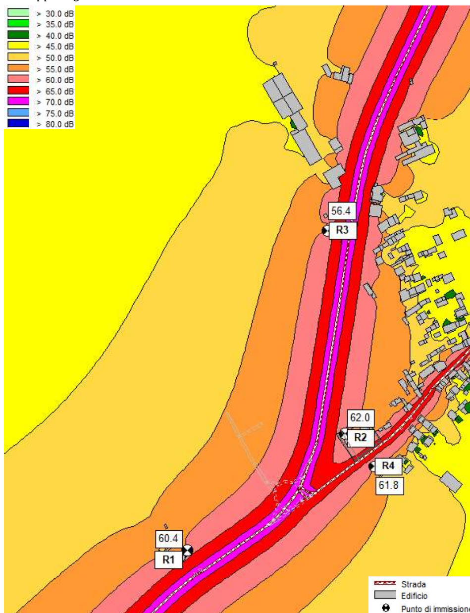
Figura 6-3 - Mappa degli isolivelli acustici DIURNI calcolata a 4 metri di altezza dal suolo – Stato di fatto.
