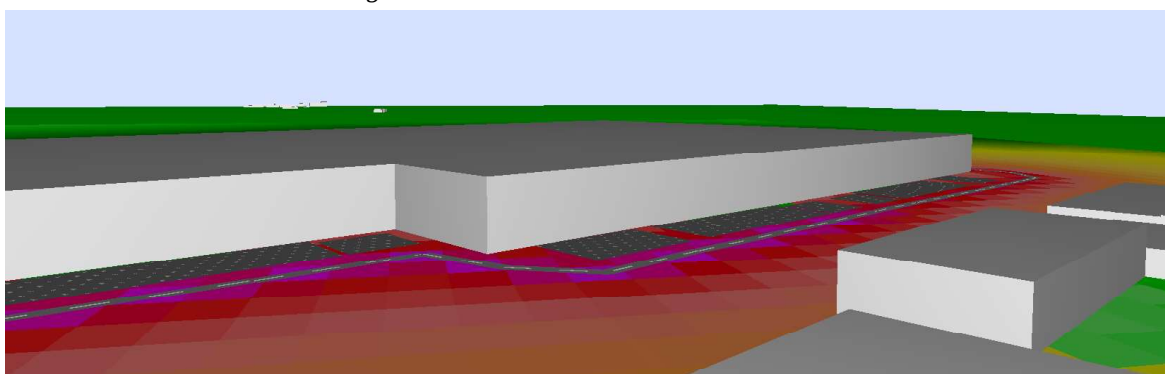
Figura 6-1 – Vista 3D del modello di calcolo.
