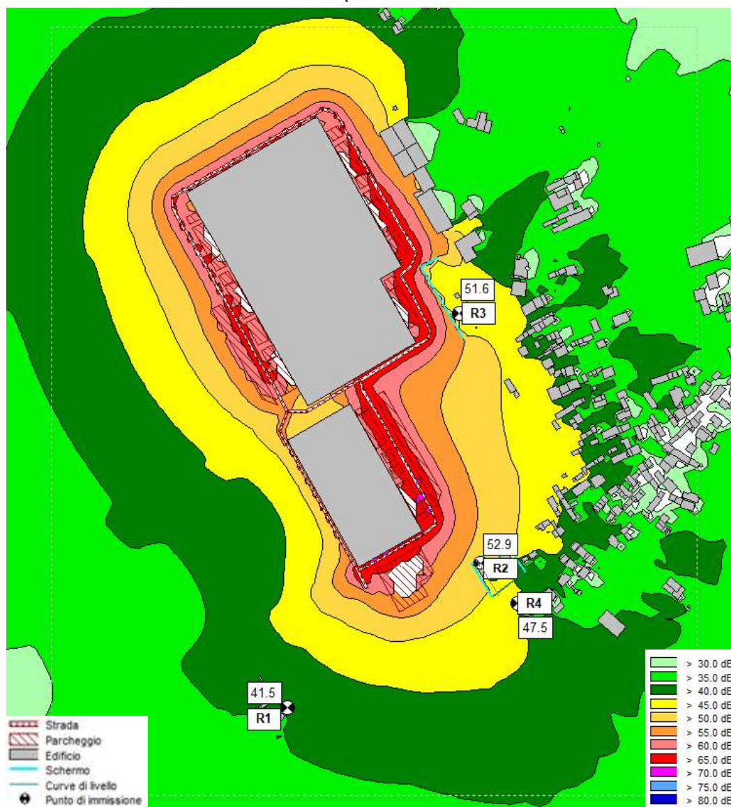
Figura 6-8 – Sorgenti interne - Mappa degli isolivelli acustici DIURNI calcolata a 4 metri di altezza dal suolo – Scenario di punta - MITIGATO
