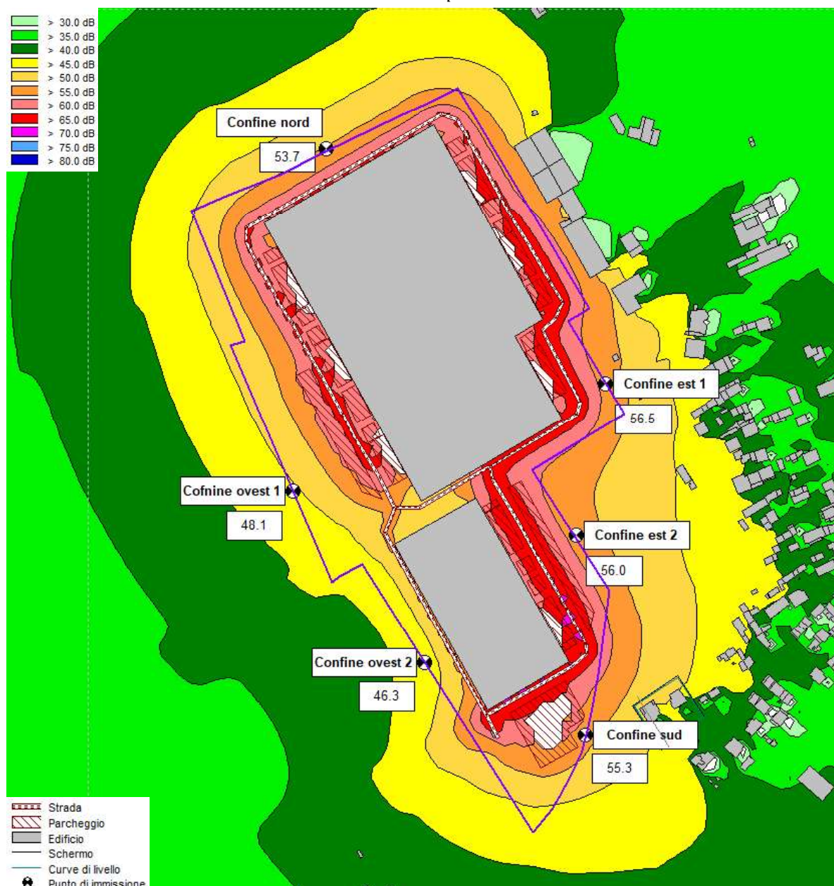
Figura 6-7 – Sorgenti interne. Mappa degli isolivelli acustici DIURNI calcolata a 4 metri di altezza dal suolo – Scenario di punta
