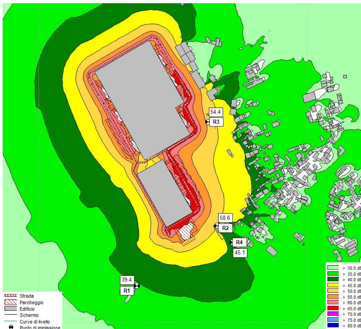
Figura 6-6 – Sorgenti interne - Mappa degli isolivelli acustici DIURNI calcolata a 4 metri di altezza dal suolo – Scenario medio
