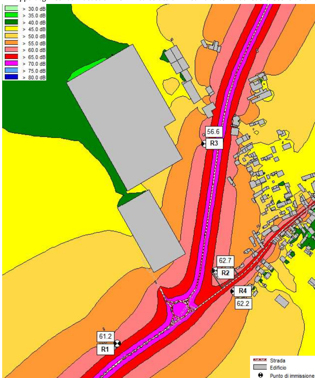
Figura 6-4 - Mappa degli isolivelli acustici DIURNI calcolata a 4 metri di altezza dal suolo. Scenario di intervento.
